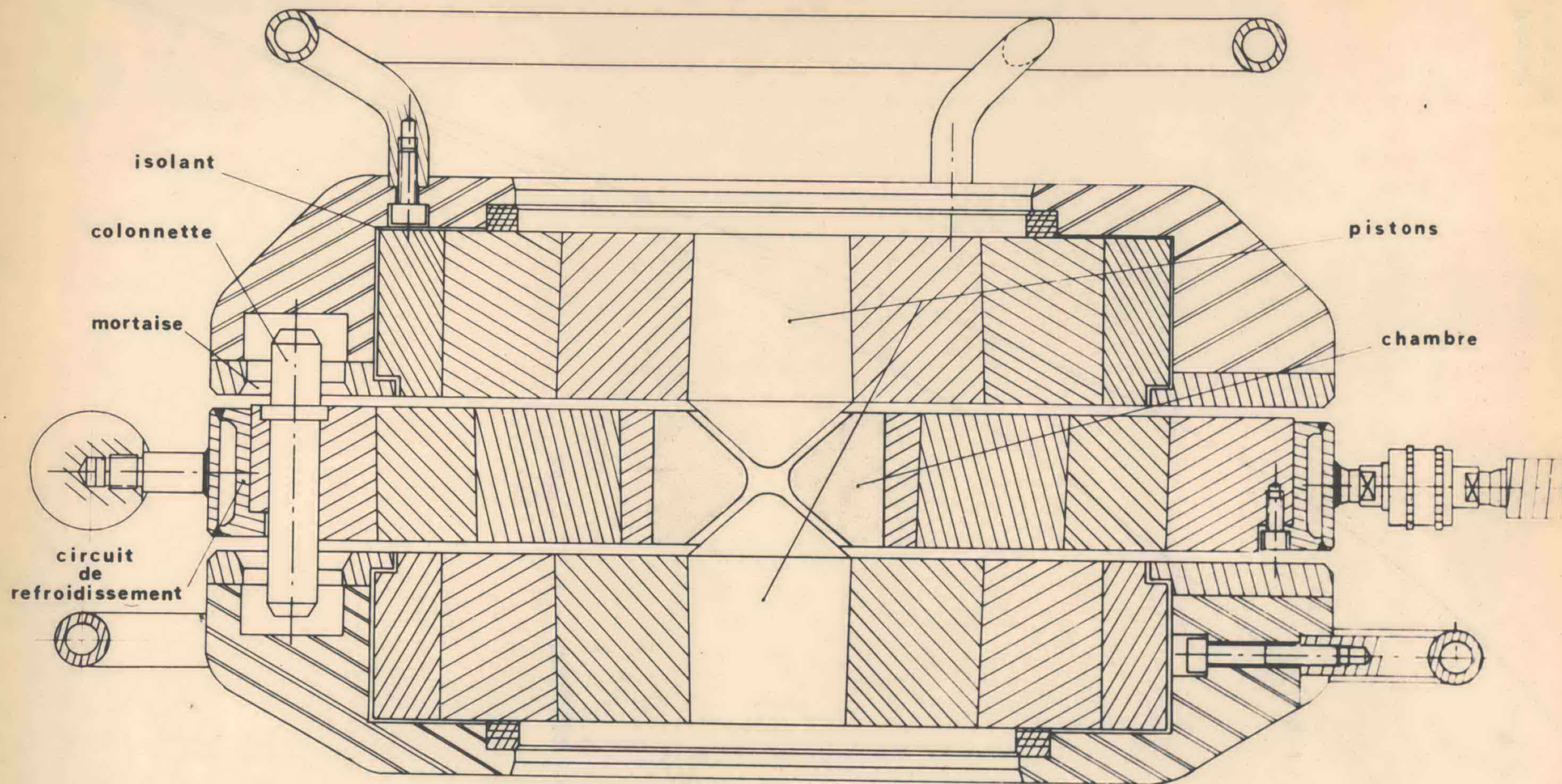
Fig III 1 ENCLUME ANNULAIRE TYPE X
