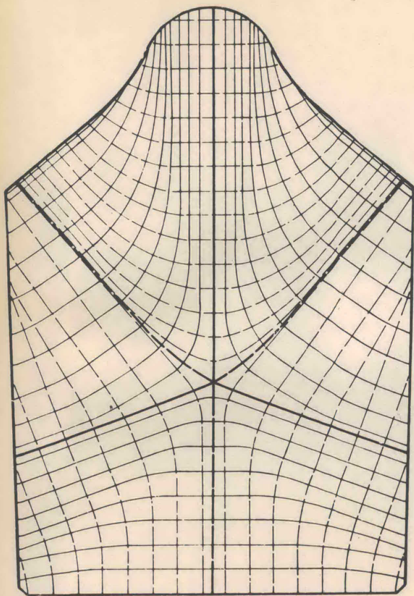
a) Piston sous charge répartie
