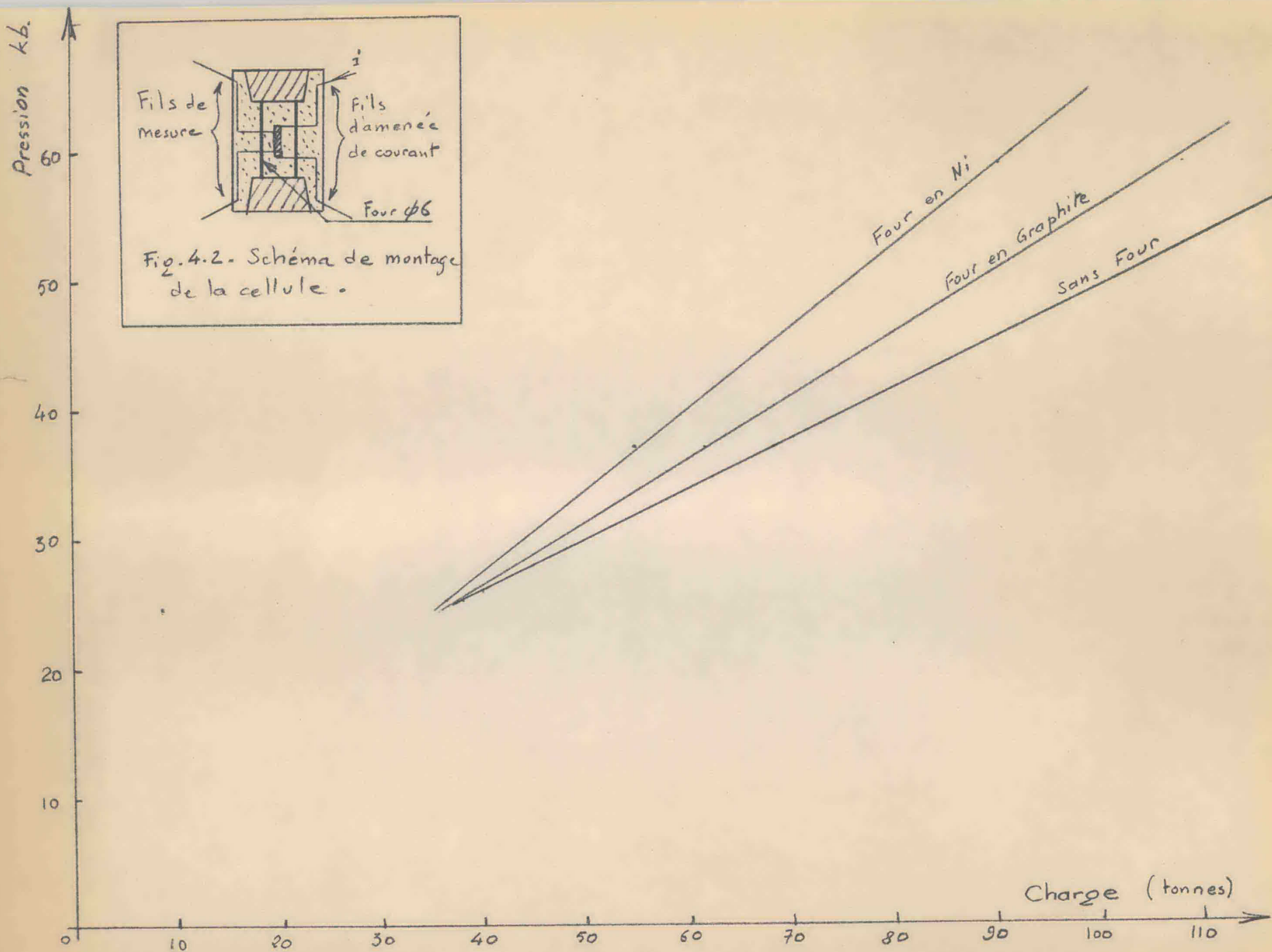
Figure 4-1. Influence de la nature du four sur la courbe d'étalonnage d'un "Belt".
