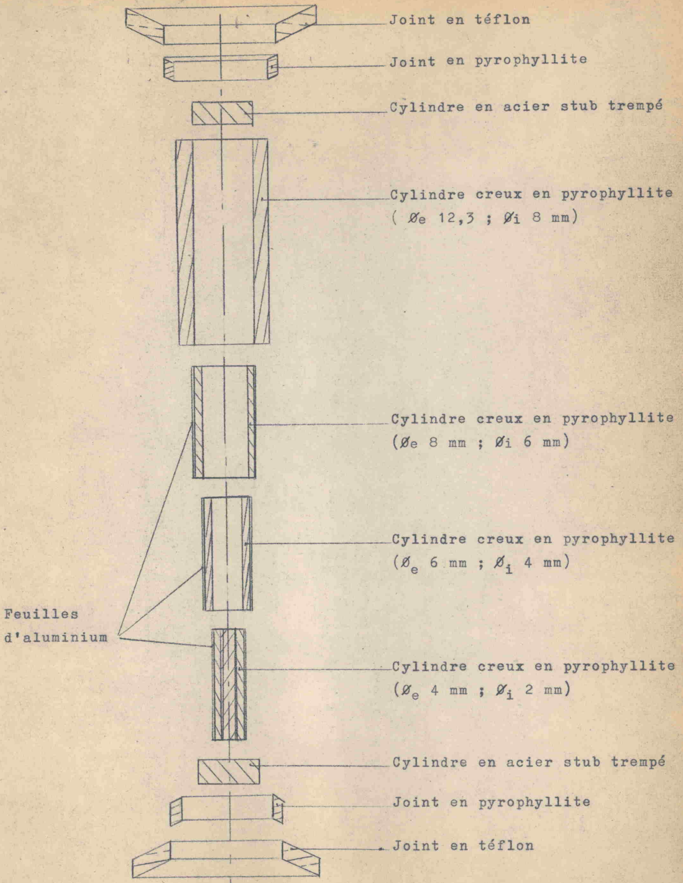
Fig. 3 -7 Montage des cylindres concentriques pour l'essai de mise en évidence des déformations.
