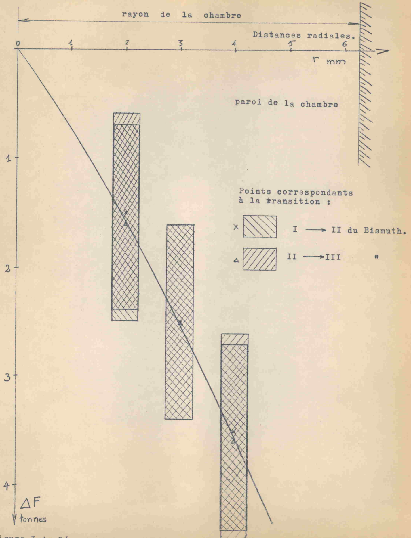
Figure 3-4; Répartition radiale de la pression dans la partie centrale de la cellule.
