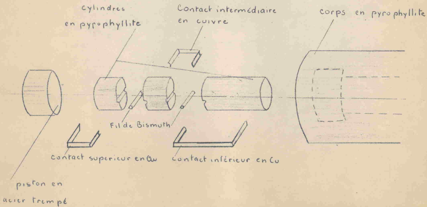
Figure 3-1. Montage utilisé pour l'étude de la répartition axiale de la pression dans la cellule.
