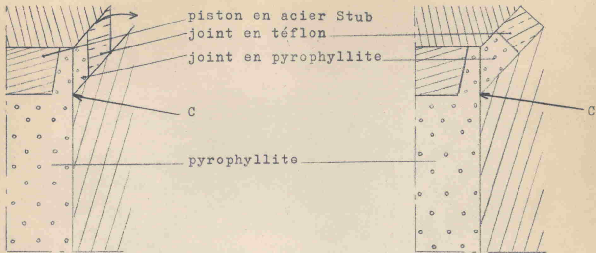
Fig. 2 -2 Joints adoptés.
