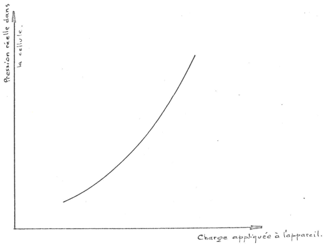
Figure 19 Allure de la courbe d'étalonnage d'une enclume de Drickamer.
