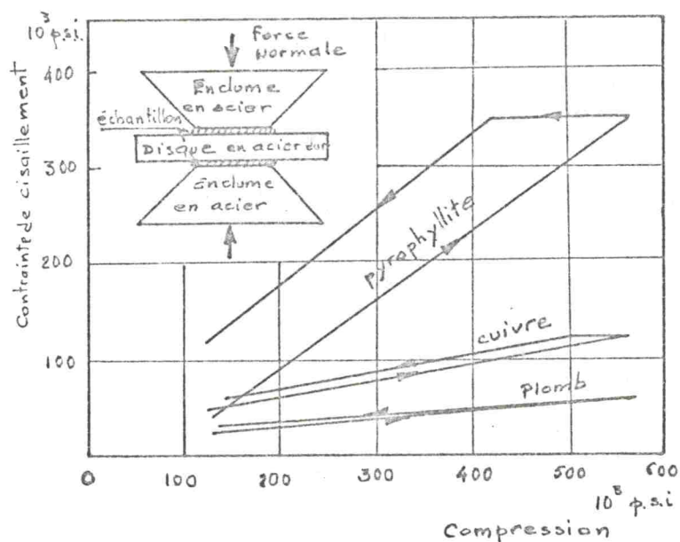
Figure 5. Contrainte de cisaillement de la pyrophyllite du cuivre et du plomb en fonction d'un effort de compression.
