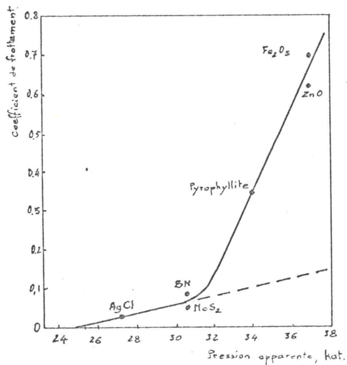
Figure 6. Pression apparente nécessaire pour obtenir la transition B_{I} \rightarrow B_{III} en fonction du coefficient de frottement interne.
