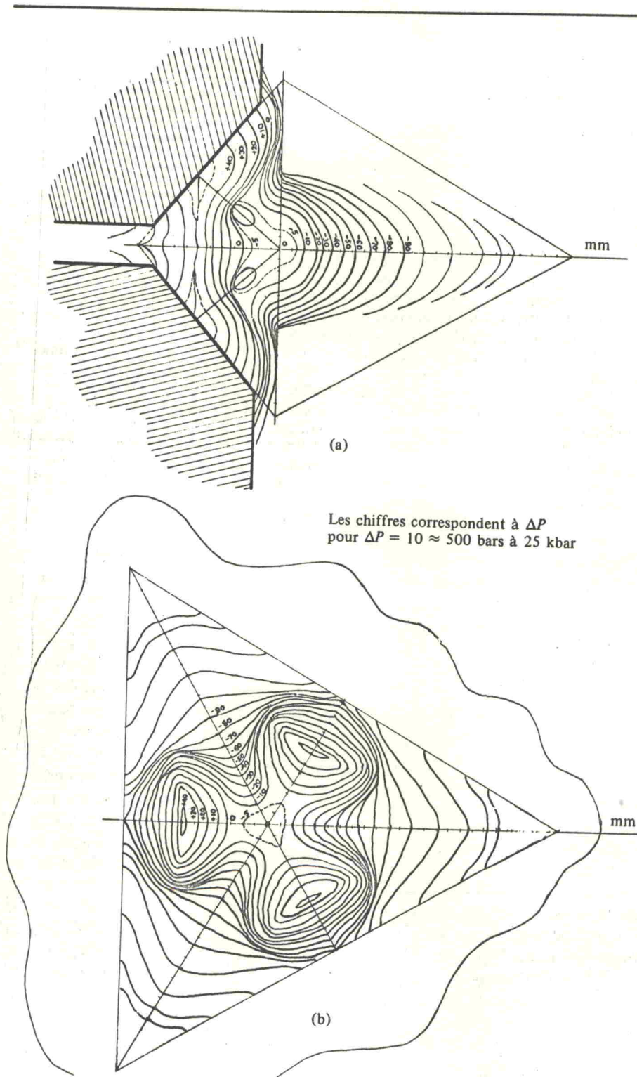
Figure 14. Tracé des isobares: (a) plan méridien, (b) plan équatorial.
