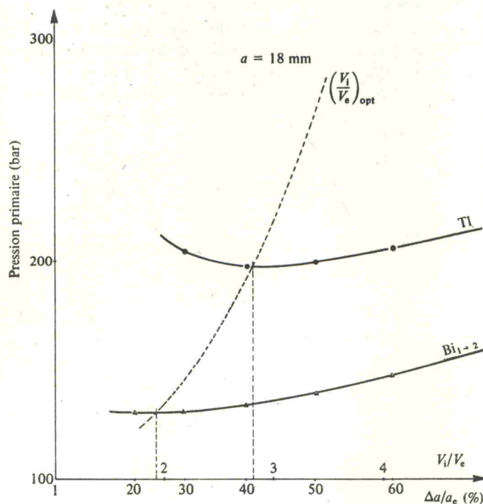
Figure 7. Optimisation du volume de l'hexaèdre initial: variation de l'optimum avec la pression pour l'enclume de a = 18 \text{ mm} .
