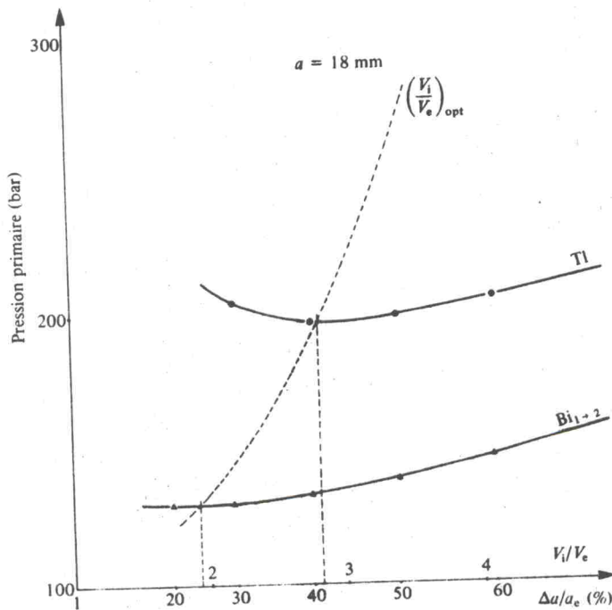
Figure 7. Optimisation du volume de l'hexaèdre initial: variation de l'optimum avec la pression pour l'enclume de a = 18 \text{ mm} .
