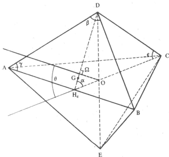
Figure 1. Hexaèdre isocèle.
