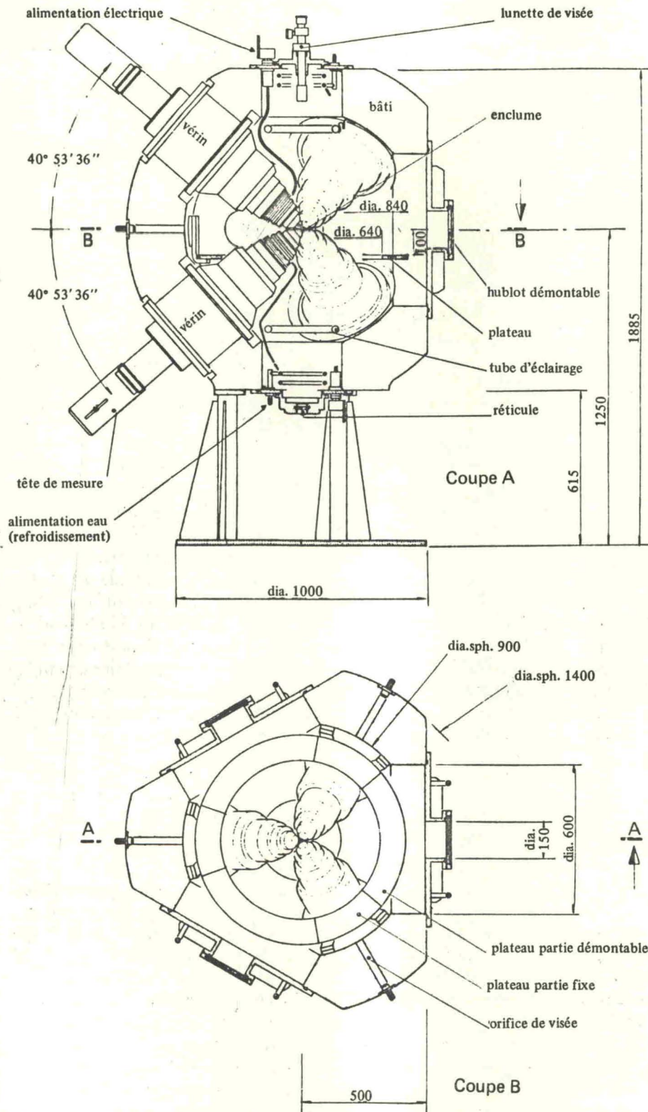
Figure 2. Schéma d'ensemble de l'enclume hexaédrique.
