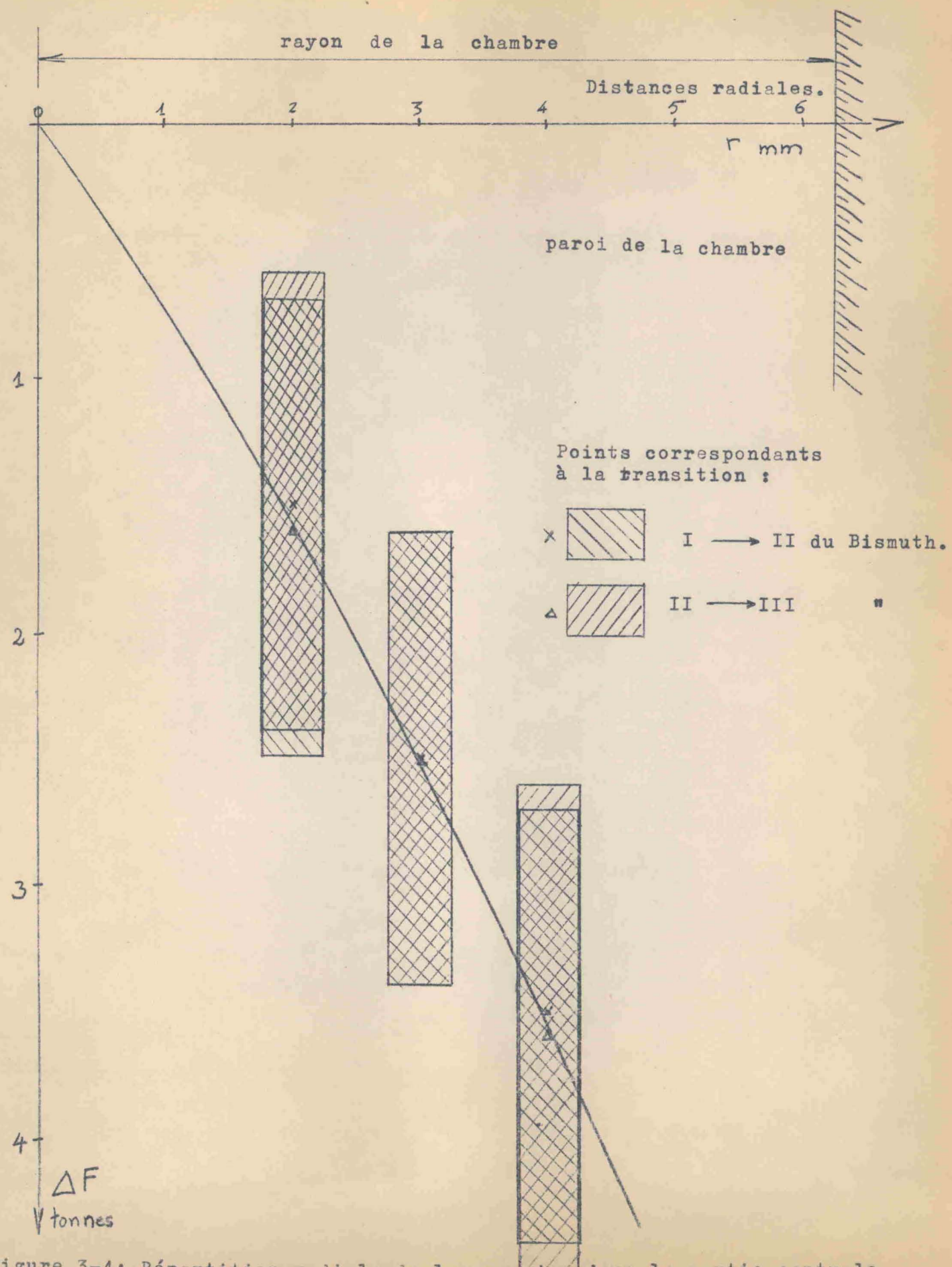
Figure 3-4; Répartition radiale de la pression dans la partie centrale de la cellule.
