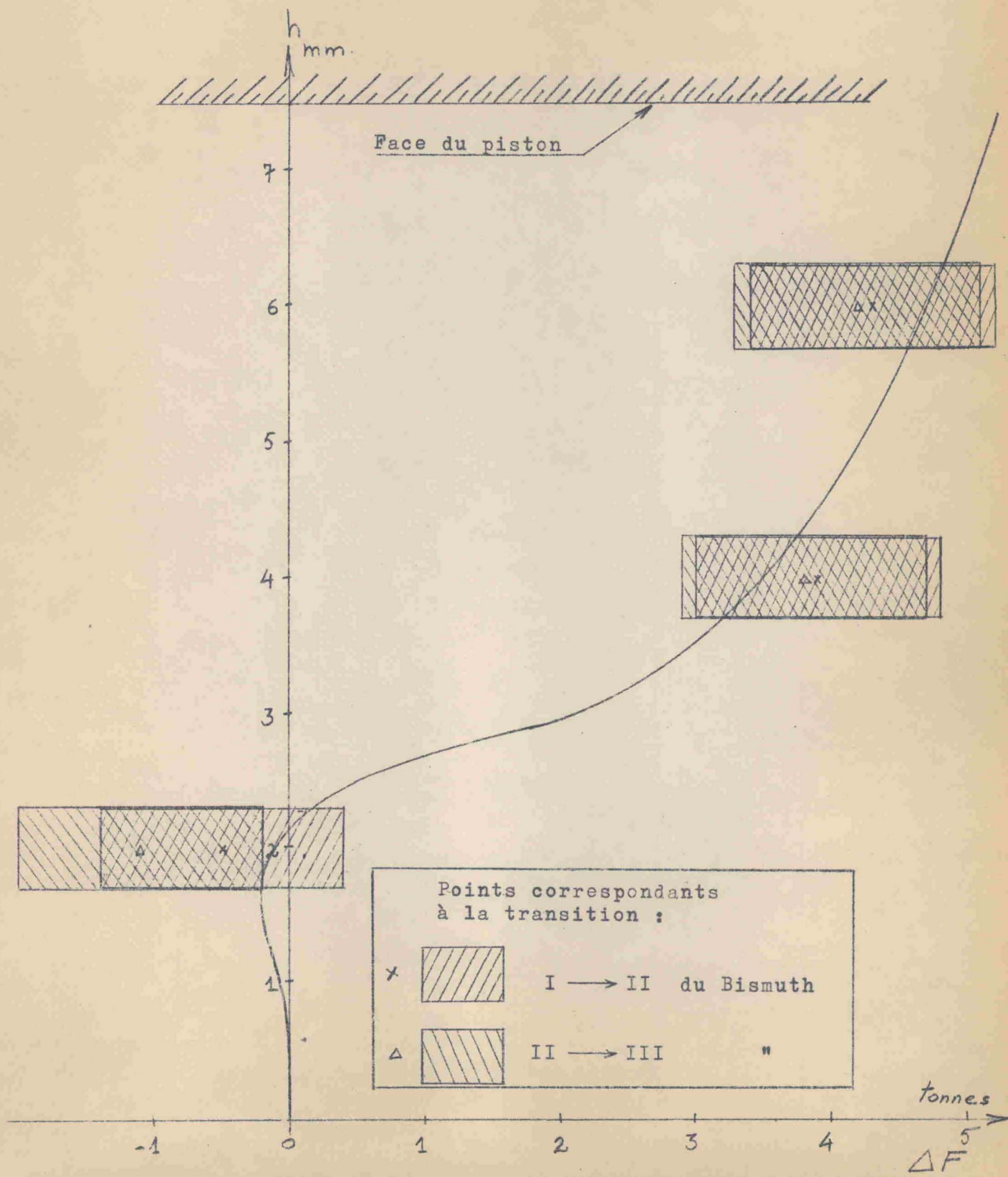
Figure 3-2 . Répartition axiale de la pression dans la cellule.
