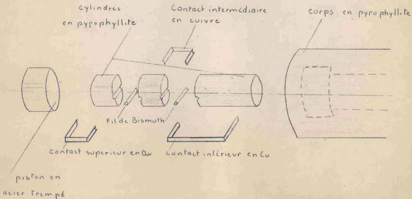
Figure 3-1. Montage utilisé pour l'étude de la répartition axiale de la pression dans la cellule.
