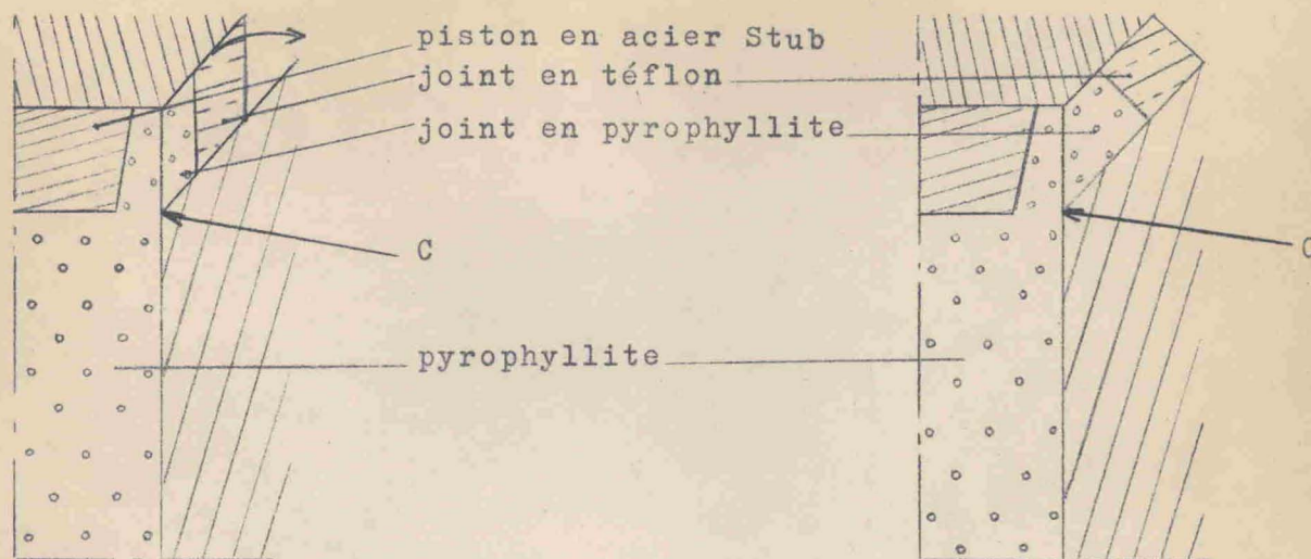
Fig. 2 -2 Joints adoptés.
