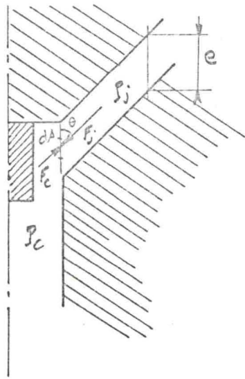
Figure 28. Jonction corps-joint
