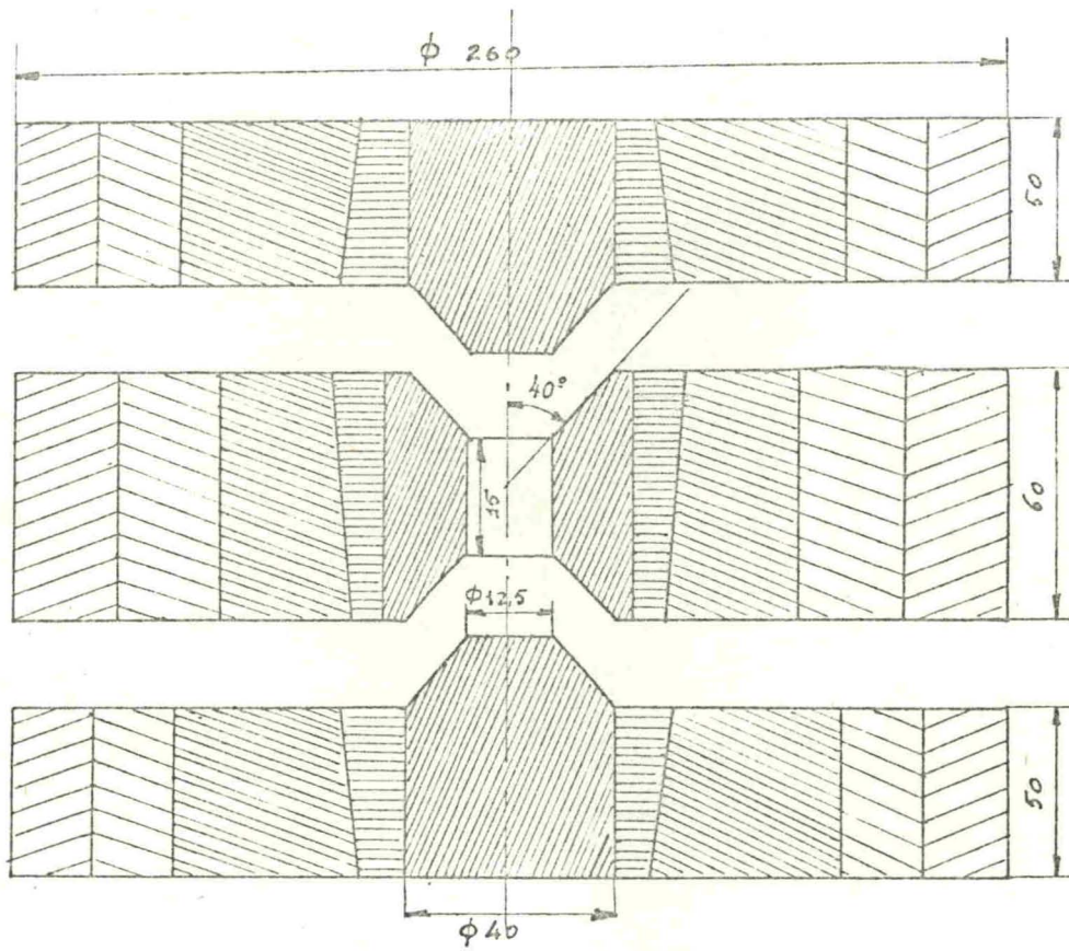
Figure 9 - Schéma du "Belt" à pistons tronconiques
