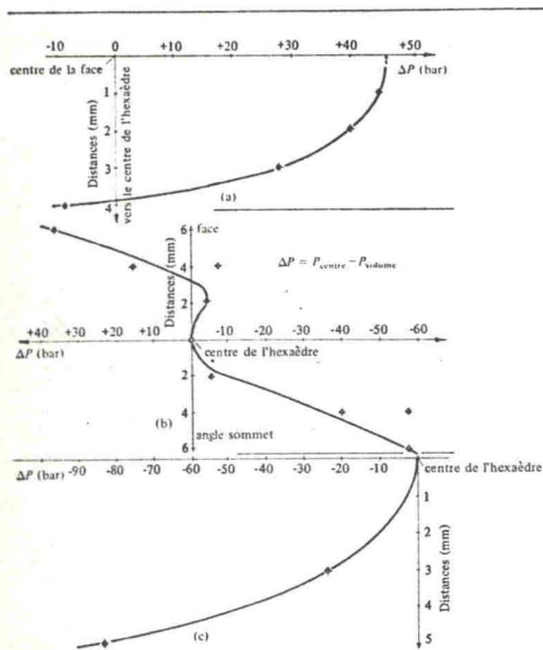
Figure 13. Répartition de la pression: (a) perpendiculairement à la face, (b) dans le plan équatorial ou de symétrie, (c) suivant l'axe de symétrie.
