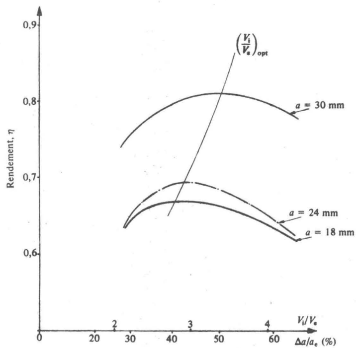
Figure 8. Variation du rendement en fonction de la taille de l'hexaèdre initial (transition du thallium).
